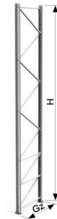
BRACING LAYOUT „ZZS”
